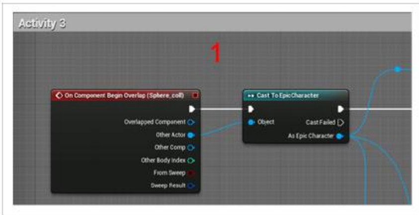
图 005a - 当玩家触碰到跳跃加成强化道具的碰撞球体后，代码就会开始运行。
